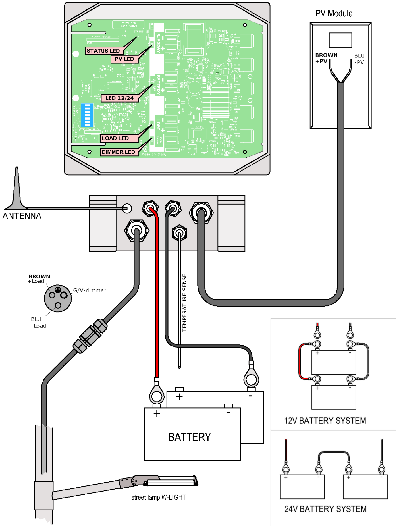
Fig. 2 Wiring scheme
